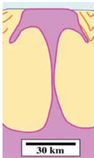
Een 5 km hoge zoutpijler in de zeebodem bij de Noordkaap.
